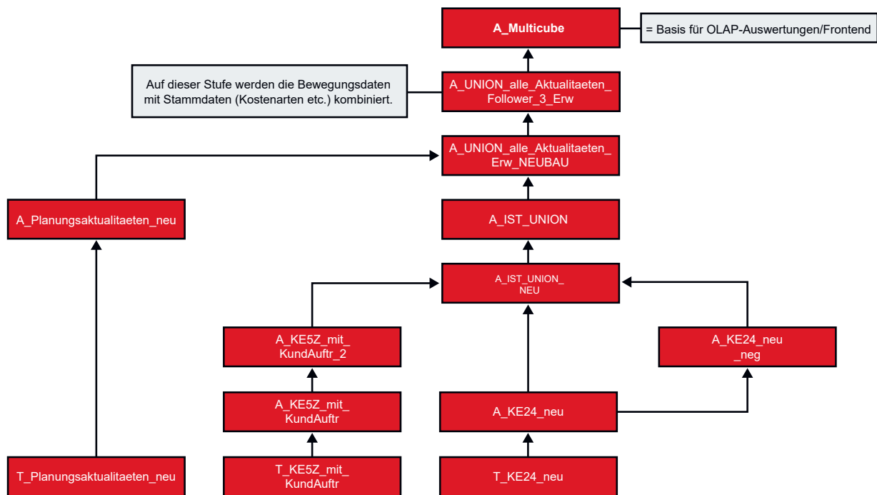
Abbildung 5: Beispiel systematischer Aufbau eines Data Warehouse
