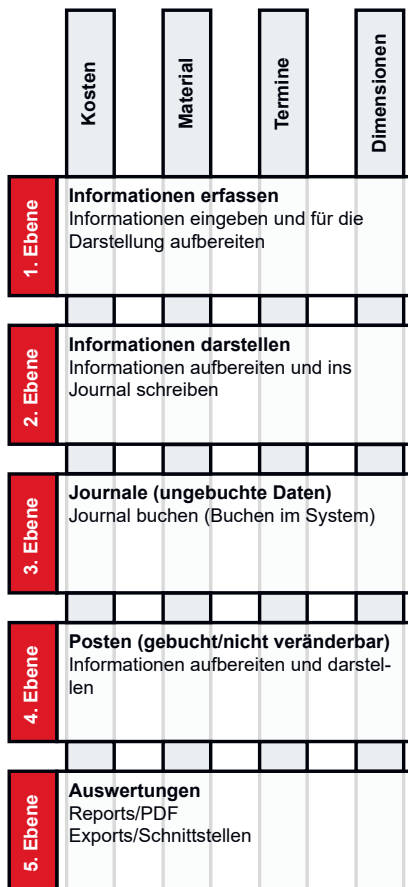
Abbildung 9: Software-Verarbeitungsebenen (Zäch, 2021)
