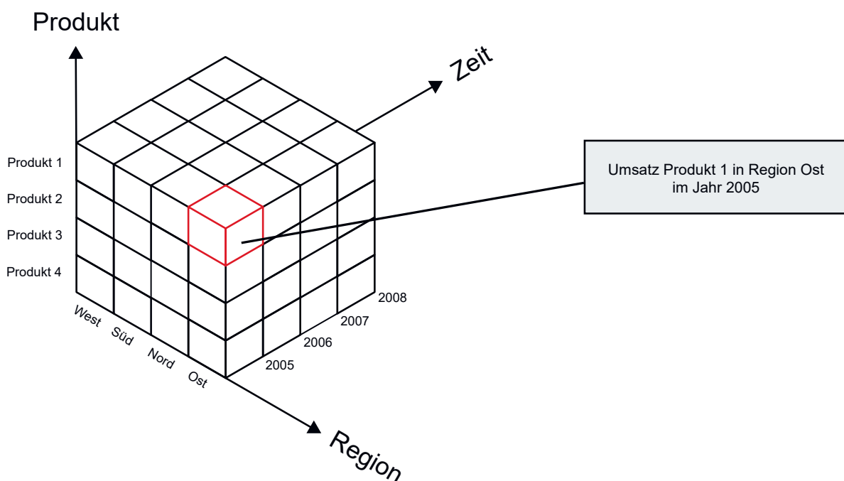
Abbildung 2: Beispiel OLAP-Cube
