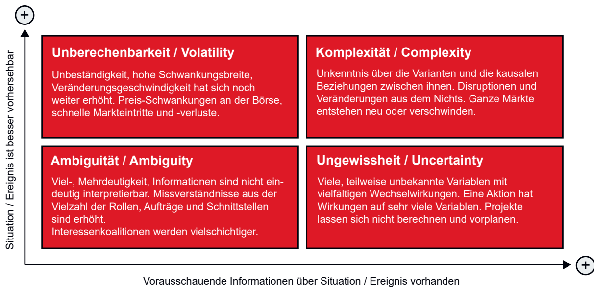
Abbildung 23: VUCA-Welt (Zäch, 2021)
