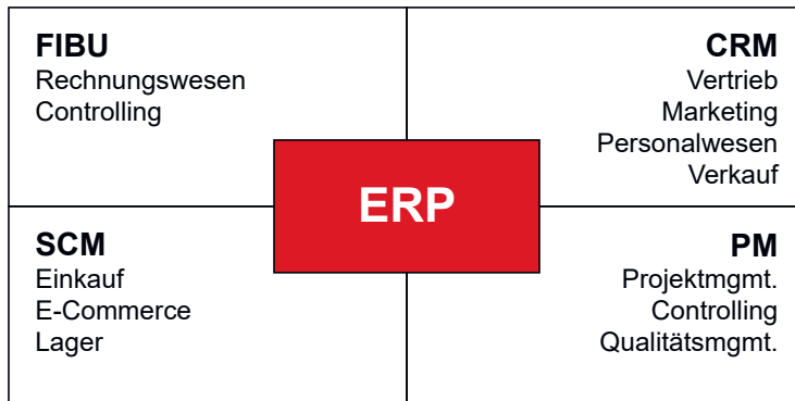
Abbildung 7: ERP-Organisation
