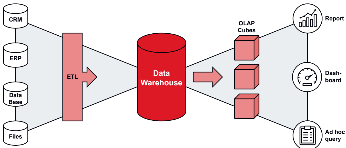
Abbildung 12: BI back/Frontend
