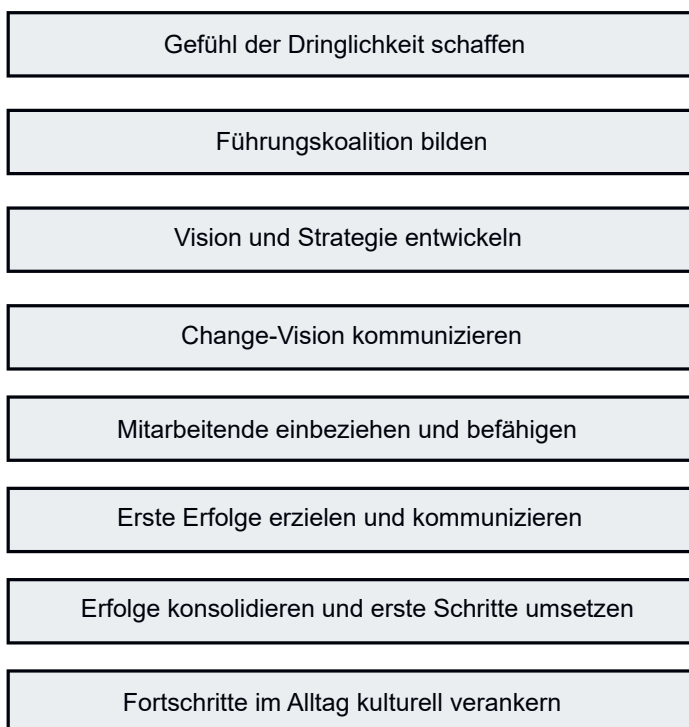
Abbildung 25: 8-Schritte-Modell (Kotter, 1996)
