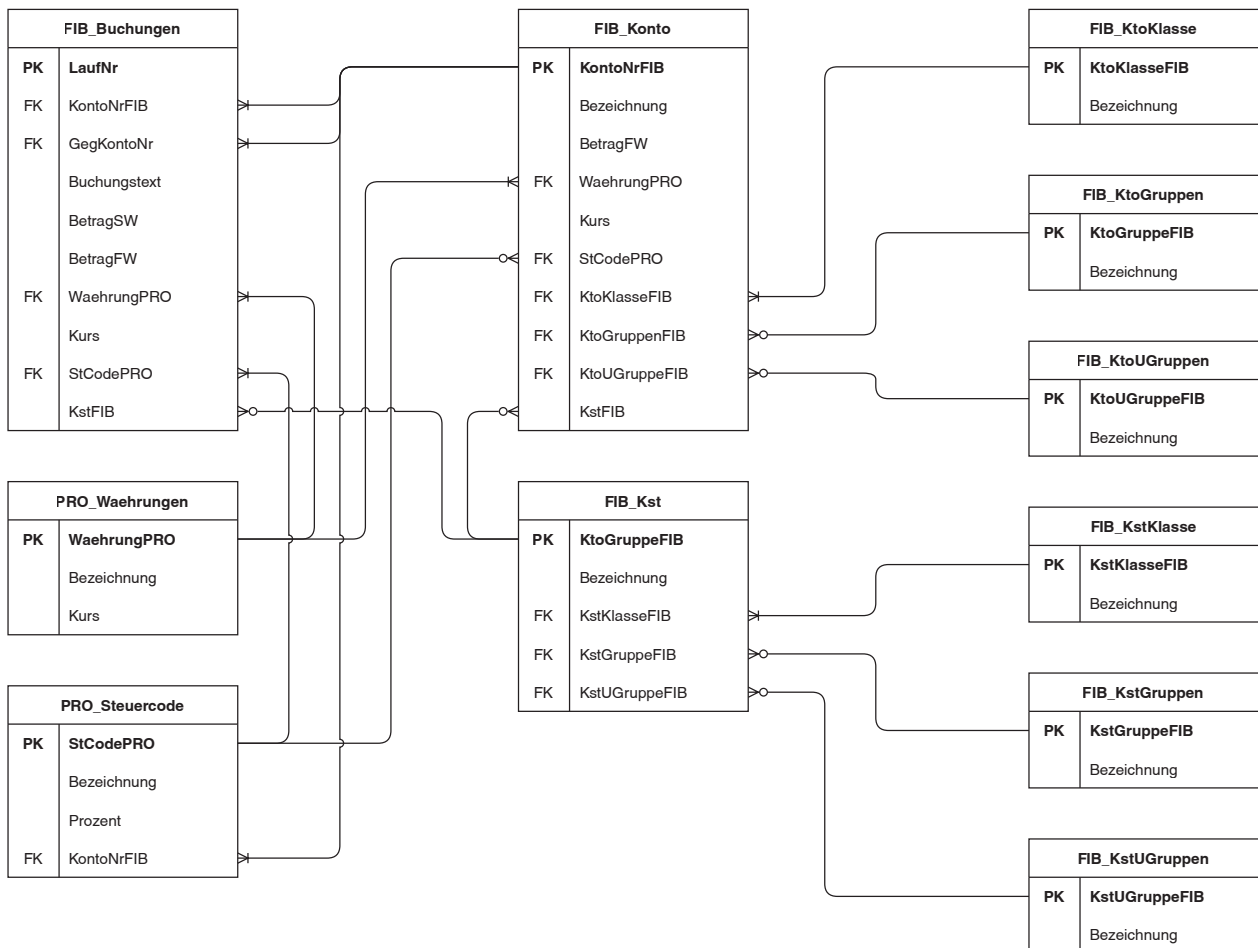
Abbildung 8: ERD-Diagramm (Proffix Px5 Finanzbuchhaltung, 2022)
